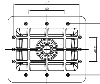
참고배면 회전 방지 돌기부 위치
