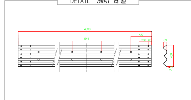
DETAIL "3WAY 레일"
