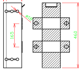
블럭아웃 SCALE:NINE
