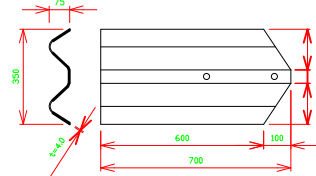
사면지주보강판 SCALE:NINE
